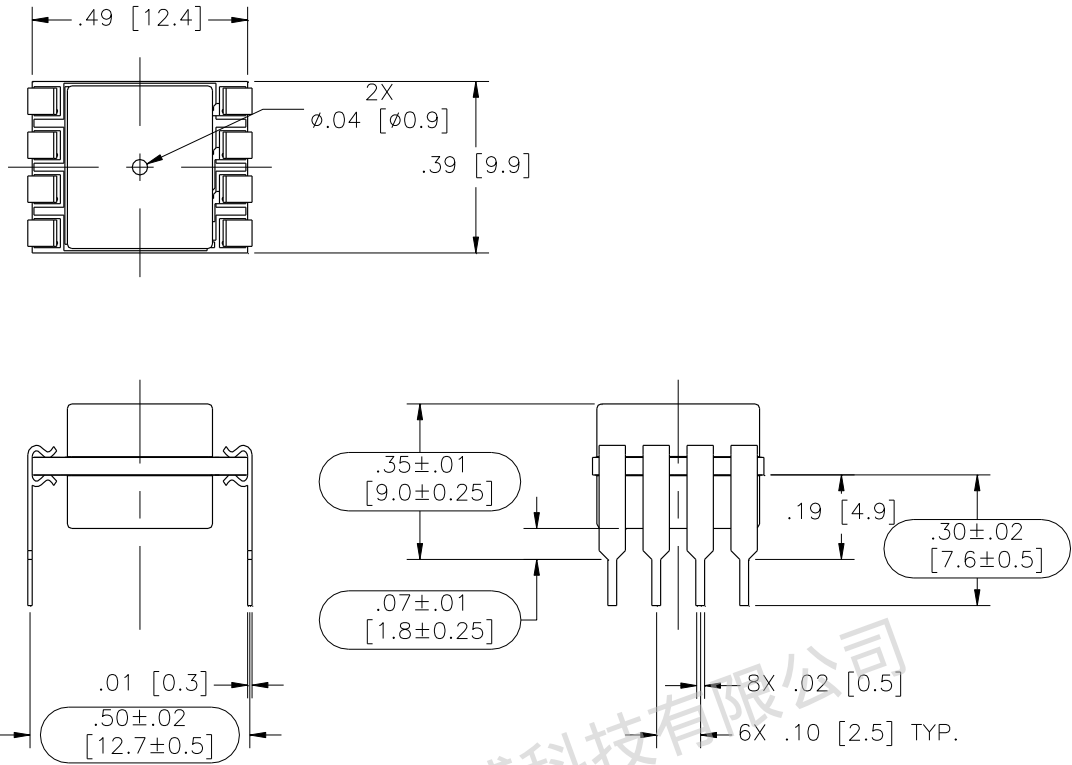
Model: MS4525DO-MMvoixxyP
