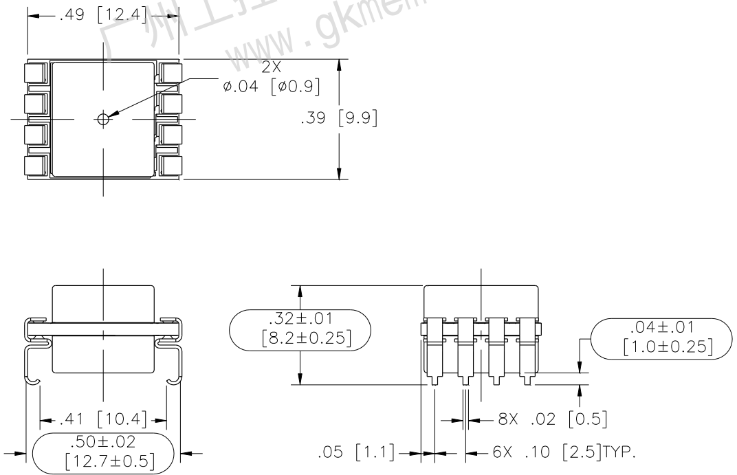
Model: MS4525DO-MMvoixxyS
